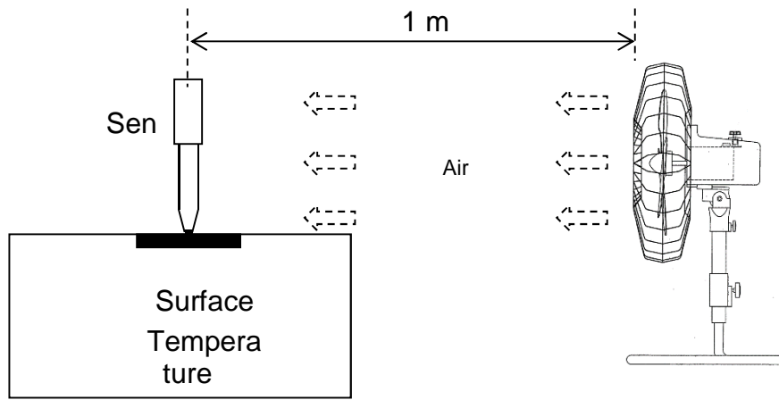
Obrázek 33 Příklad jednoduché úlohy pro měření vlivu proudění vzduchu na teplotu měřenou povrchovým teploměrem
