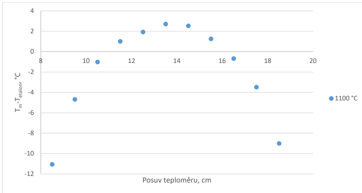
Obrázek 1: Teplotní rozložení v přenosné pídce
