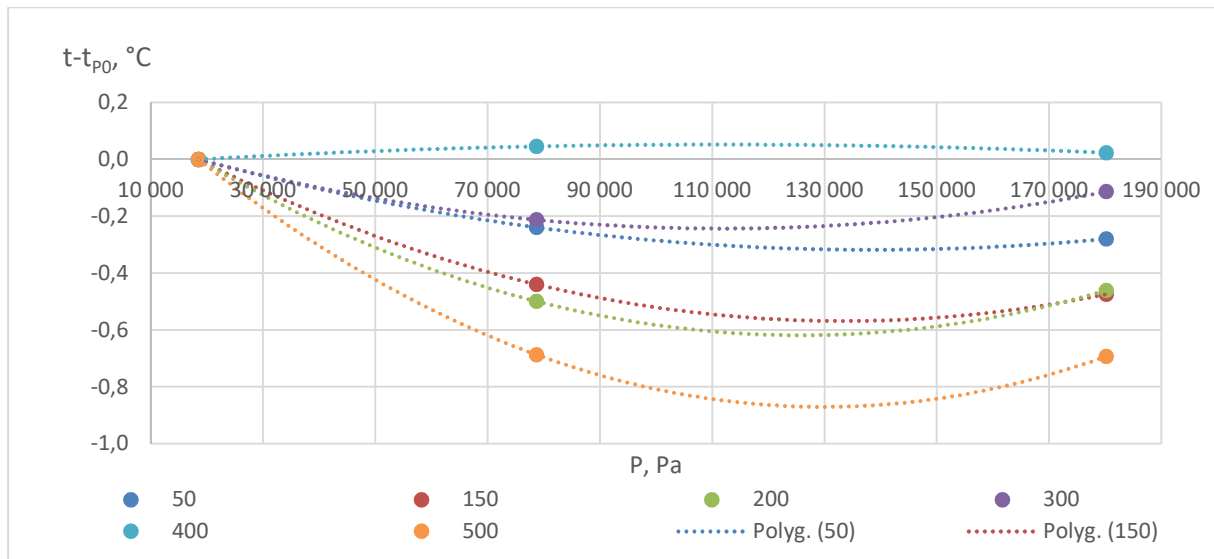
Obrázek 39 Příklad rozdílu mezi teplotou změřenou při přtlaku zvýšeném a při statickém přtlaku (hmotou sondy), pro různé jmenovité teploty, sonda č. 3
