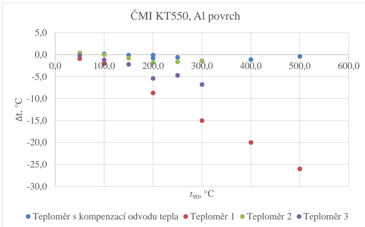
Obrázek 26 Rozdíl mezi teplotou změřenou povrchovým teploměrem a termoelektrickým snímačem teploty 1 mm pod povrchem
