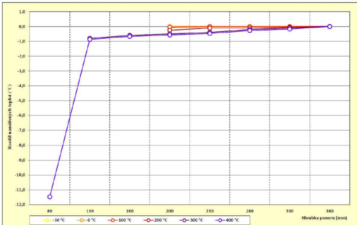
Obrázek 17: Typická chyba ponoru IPRT v kapalinové lázni
