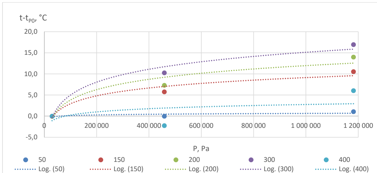
Obrázek 37 Příklad rozdílu mezi teplotou změřenou při přtlaku zvýšeném a při staticém přtlaku (hmotou sondy), pro různé jmenovité teploty, sonda č. 1
