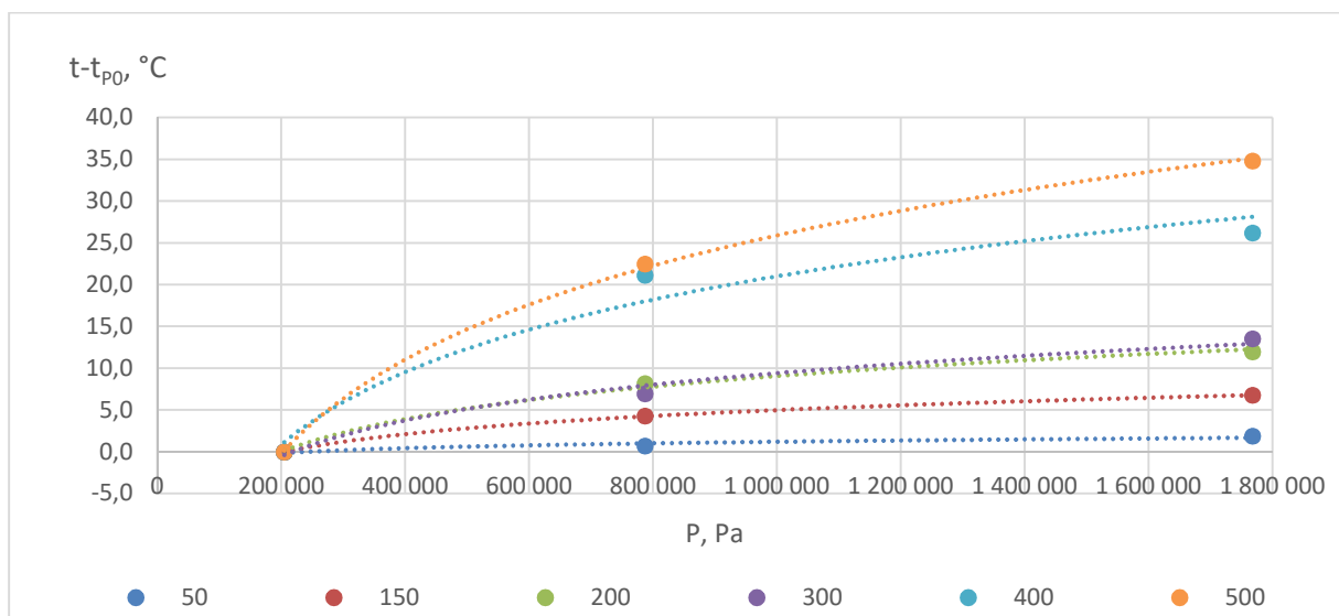
Obrázek 38 Příklad rozdílu mezi teplotou změřenou při přtlaku zvýšeném a při staticém přtlaku (hmotou sondy), pro různé jmenovité teploty, sonda č. 2
